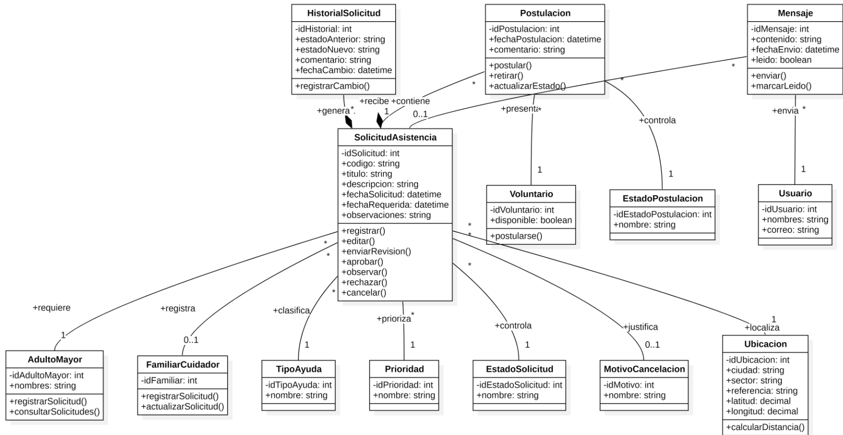
Ilustración 7 Diagrama de solicitudes y colaboración
