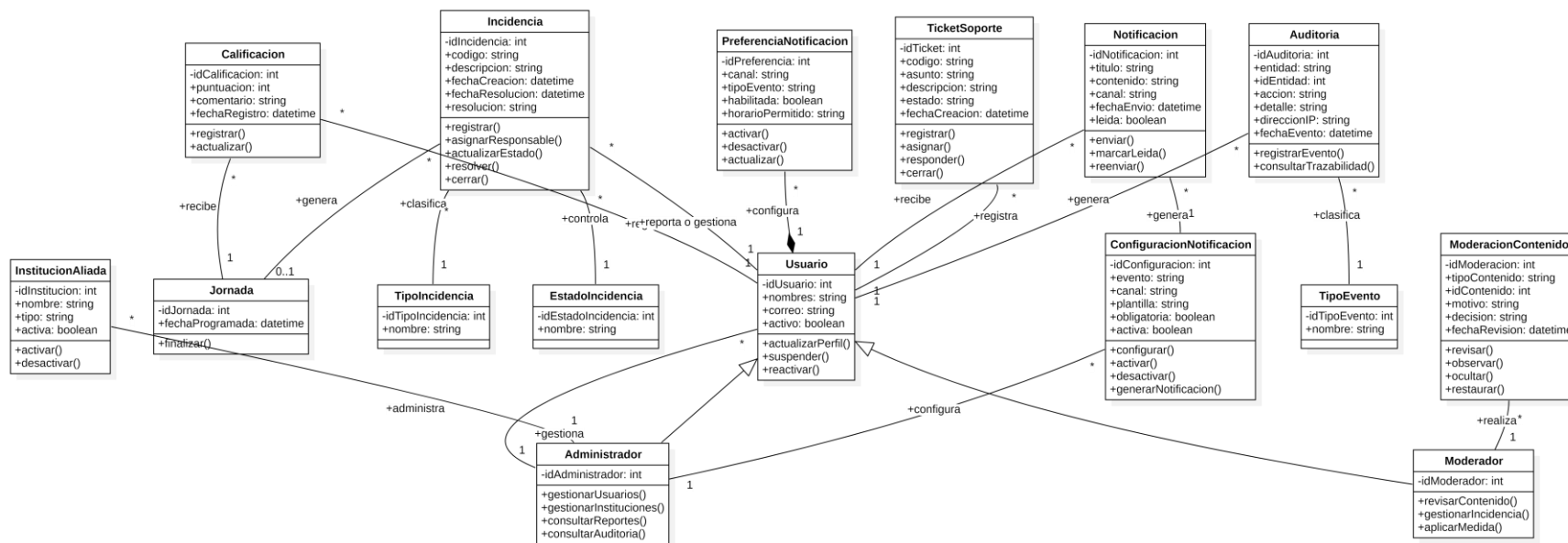
Ilustración 9 Diagrama de evaluación, administración y control
