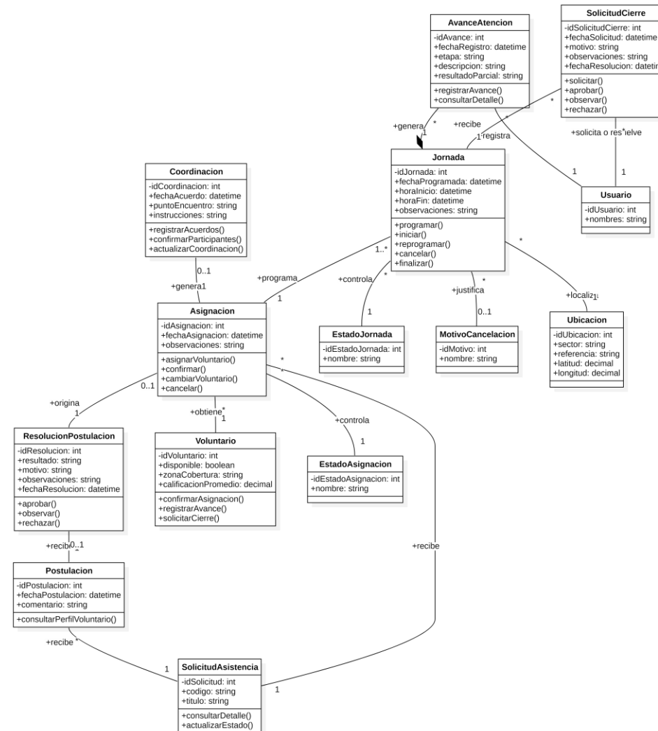
Ilustración 8 Diagrama de coordinación y atención.
