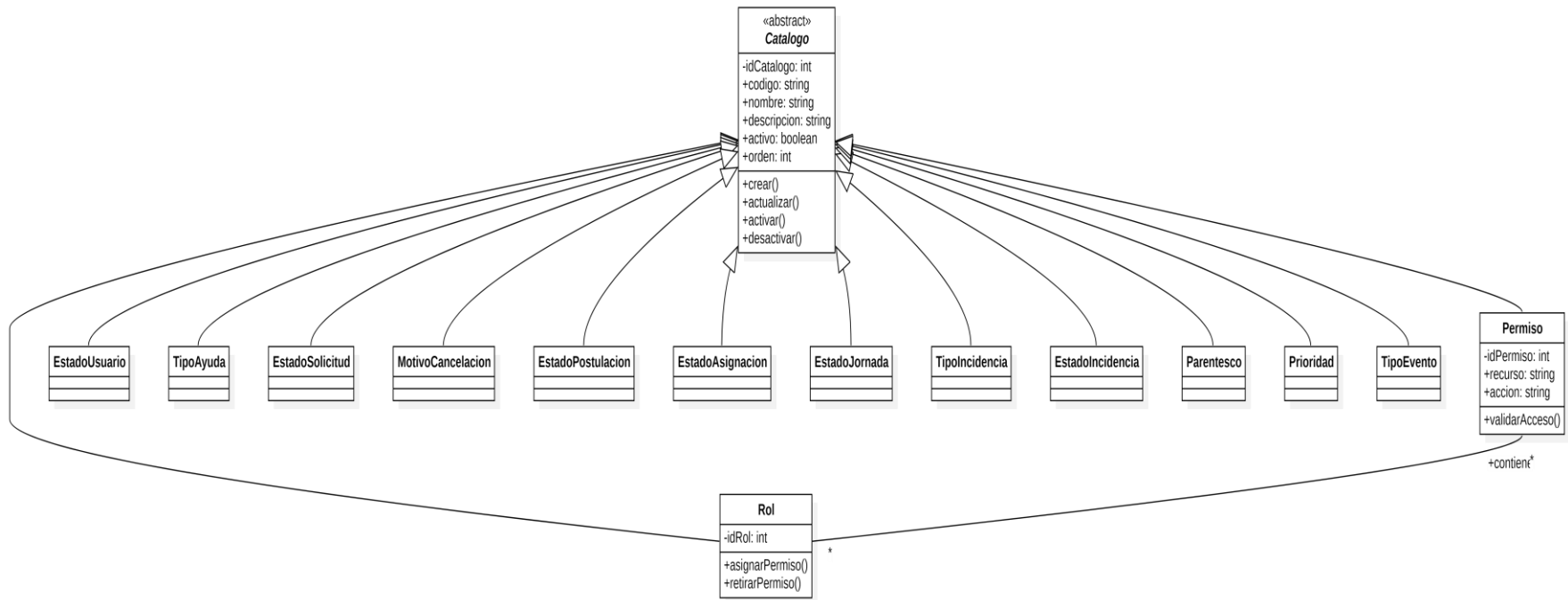
Ilustración 5 Diagrama de catálogos
