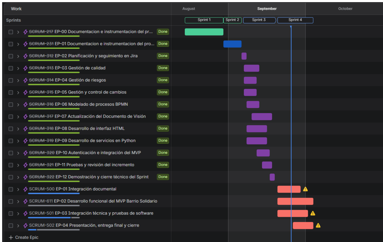
Ilustración 77 Cronograma JIRA
