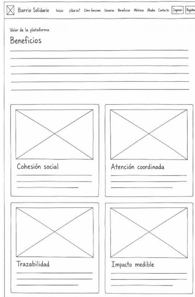
Ilustración 17 Wireframe página beneficios
