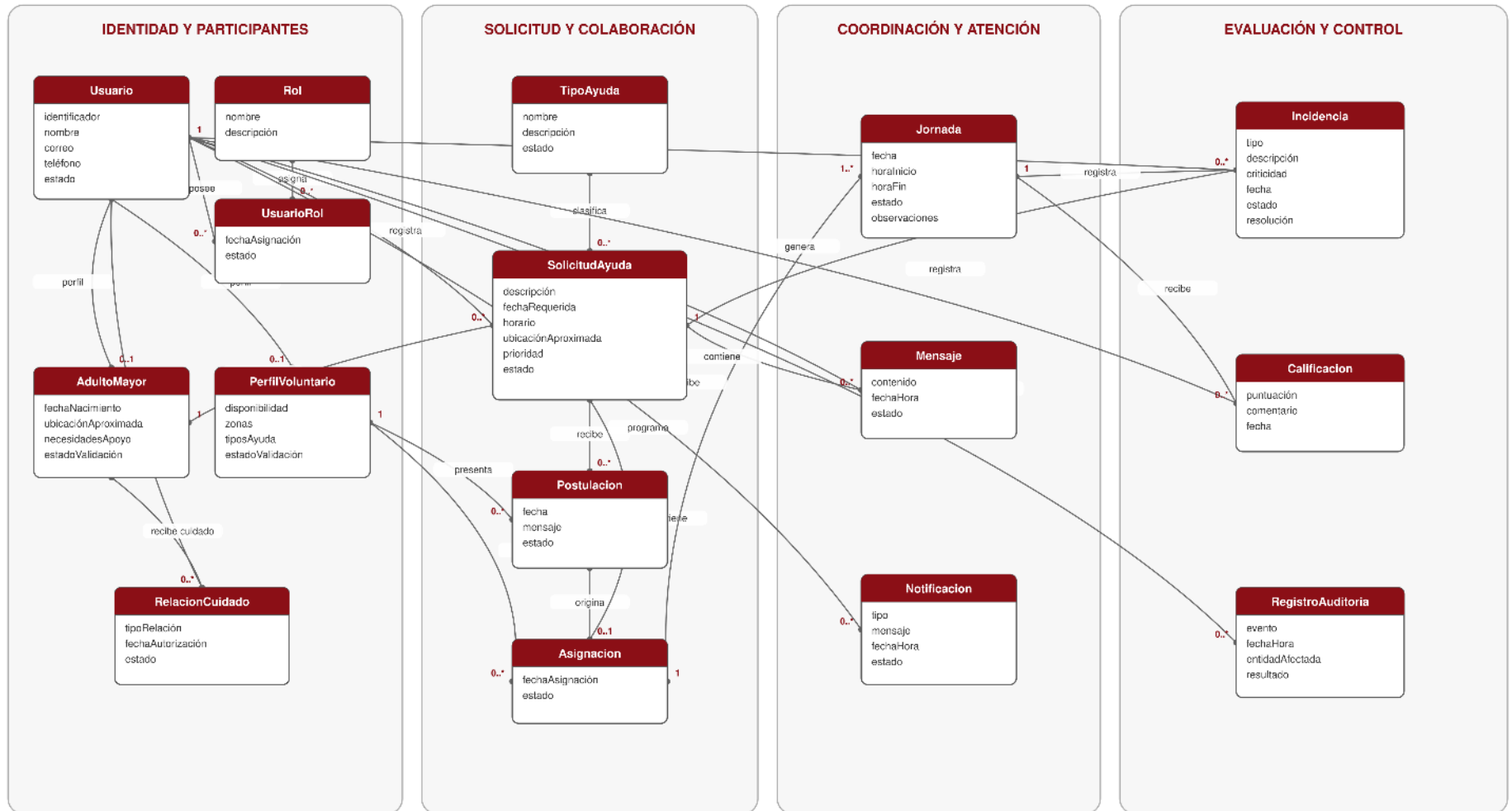
Ilustración 2 Diagrama de dominio
