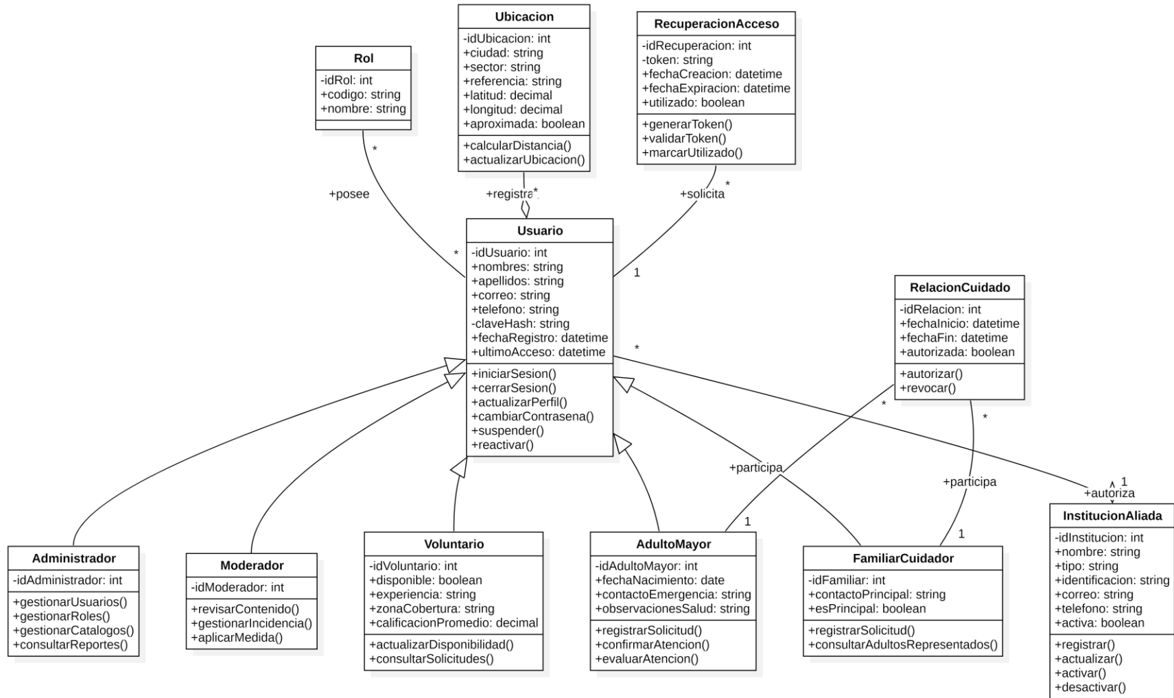
Ilustración 6 Diagrama de identidad y participantes
